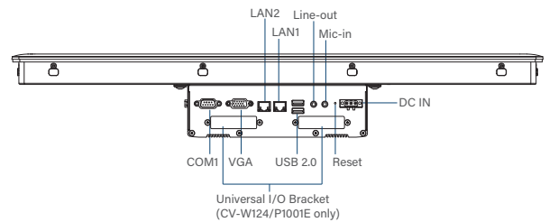
Right I/O
