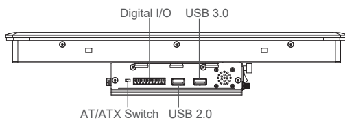
Left I/O
